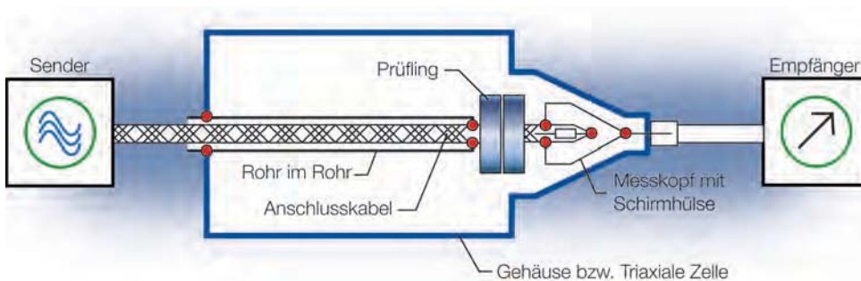
Bild 12: Triaxiale Zelle, Prinzip
