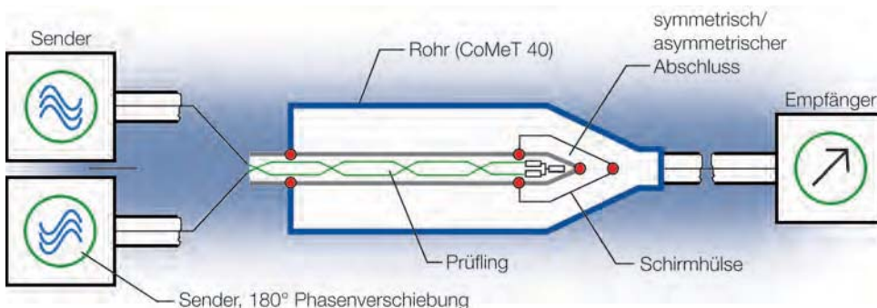
Bild 4: Messen der Kopplungsdämpfung
