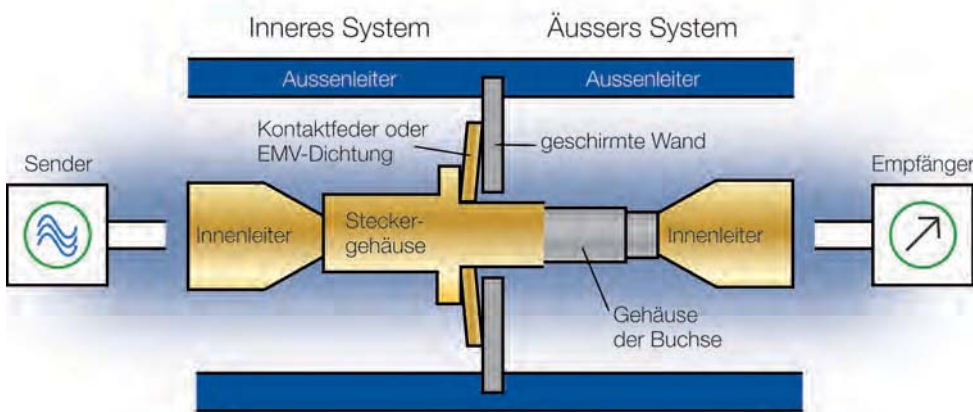
Bild 16: Messen von EMV-Dichtungen und Durchführungen, Prinzipdarstellung
