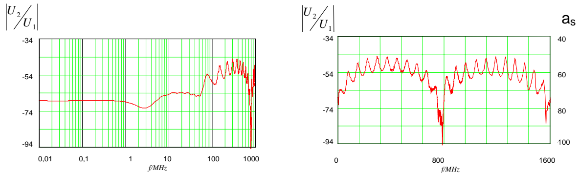
Bild 12: Frequenzgang des logarithmischen Spannungsverhältnis |U_2/U_1| in dB (linke Skala) und Schirmdämpfung a_s (rechte Skala) des Kabeltyp HF 75 1,0/4,8 02YCY, r_1=2,3 , |\Delta v/v_1|=24\% , Wirklänge l = 2 m
