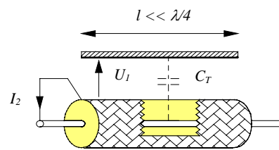
Bild 2: Definition des Durchgriffsleitwertes
