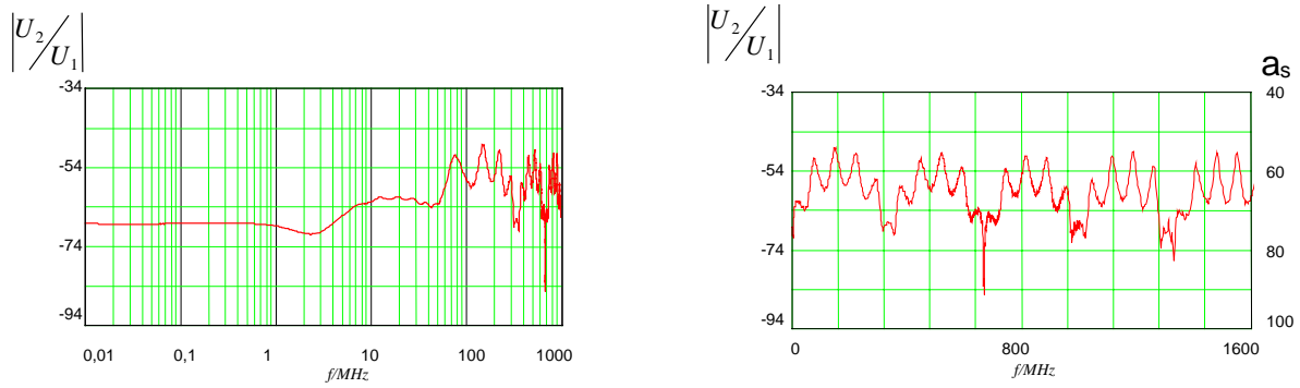
Bild 11: Frequenzgang des logarithmischen Spannungsverhältnis |U_2/U_1| in dB (linke Skala) und Schirmdämpfung a_s (rechte Skala) des Kabeltyp HF 75 0,7/4,8 2YCY, r_1=2,3 , |\Delta v/v_1|=45\% , Wirklänge l = 2 m
